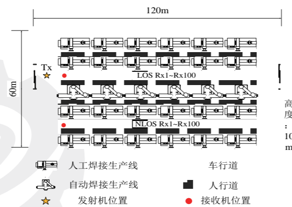
图 2-7 焊接车间 LOS 与 NLOS 测量环境
